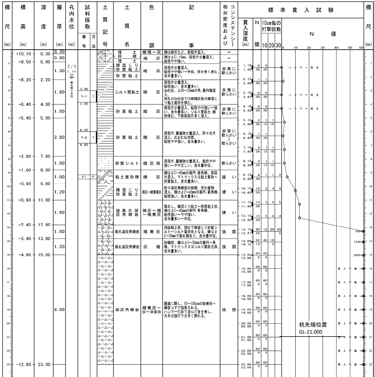
柱状図
