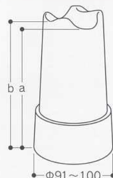
Aタイプ標準図
